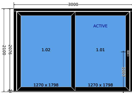
Buitenaanzicht
